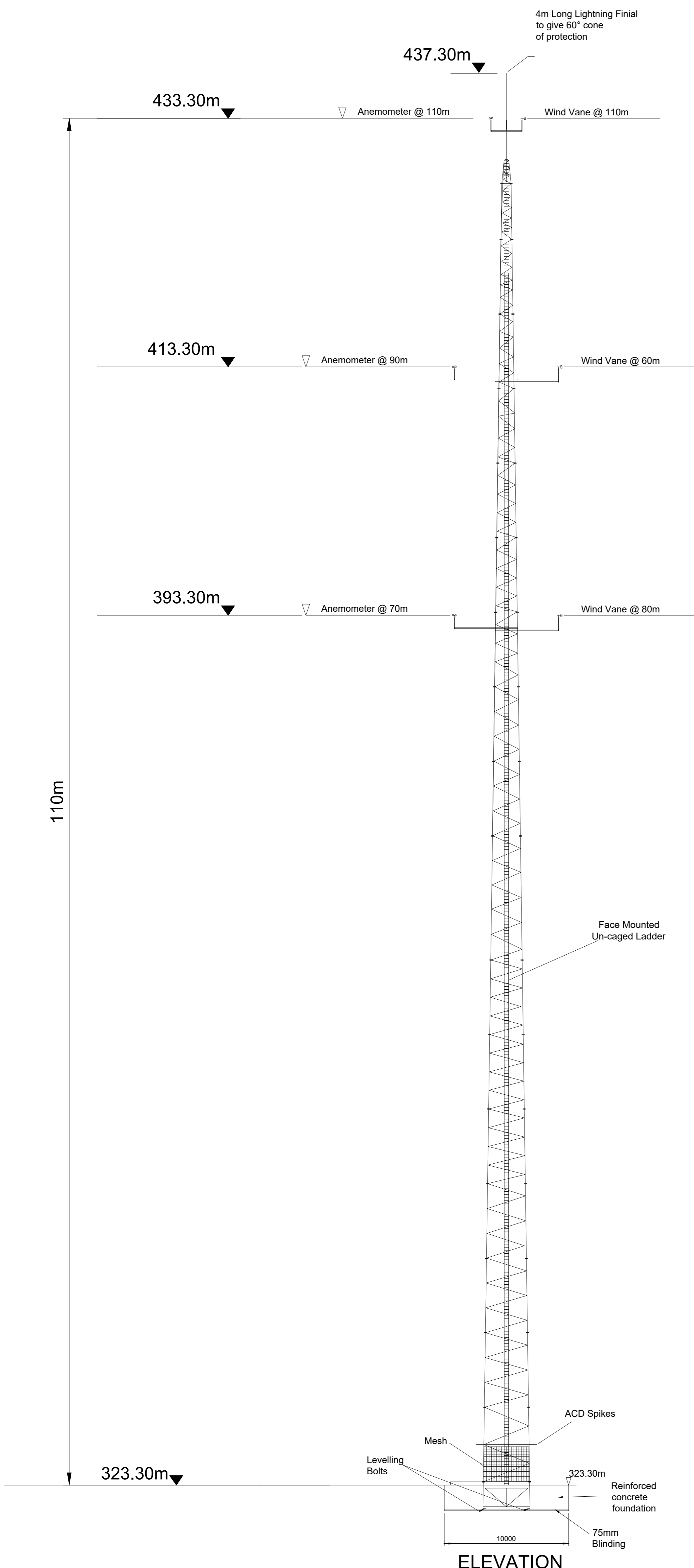
ELEVATION
